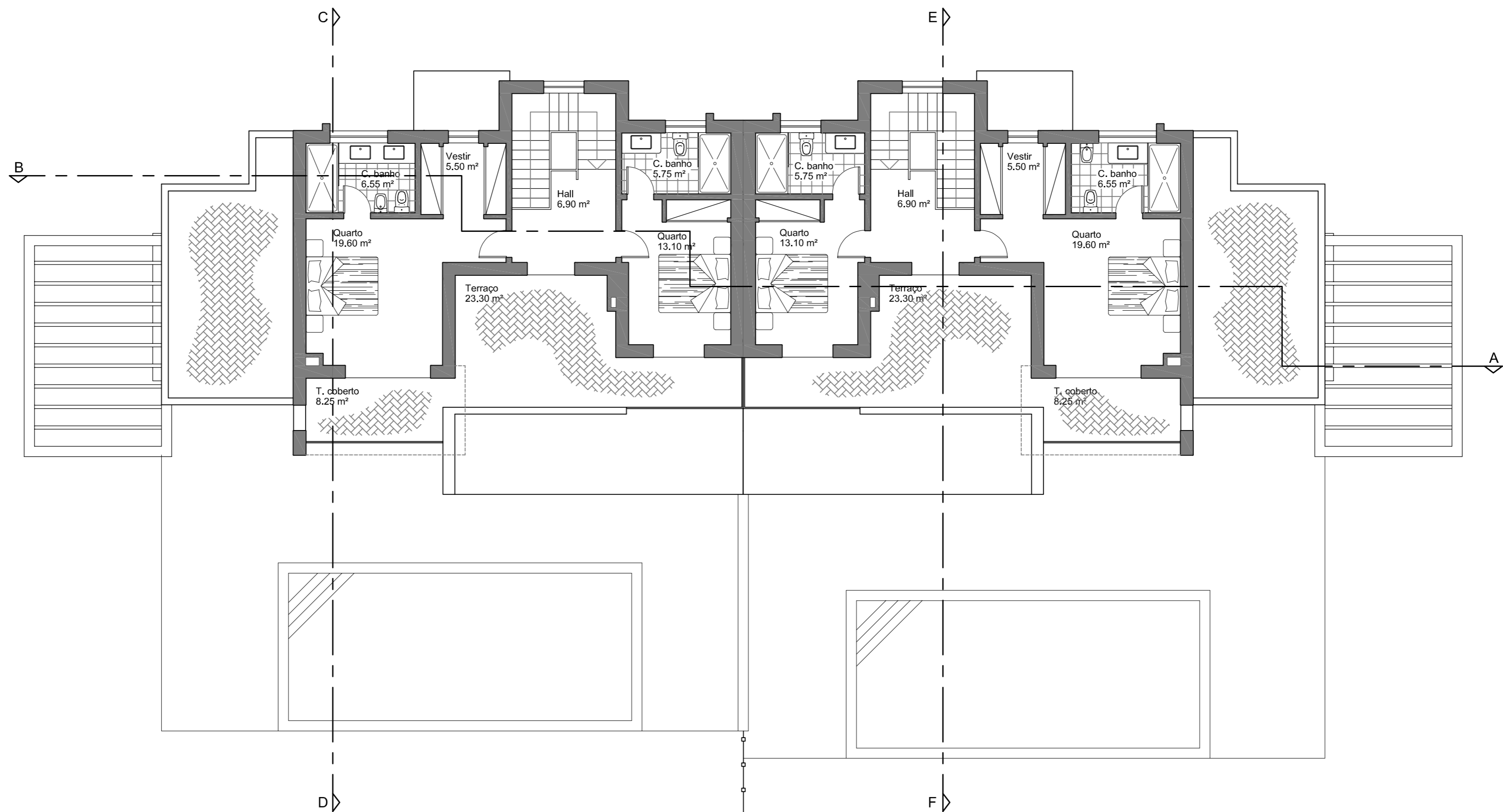
PLANTA DO 1º ANDAR
