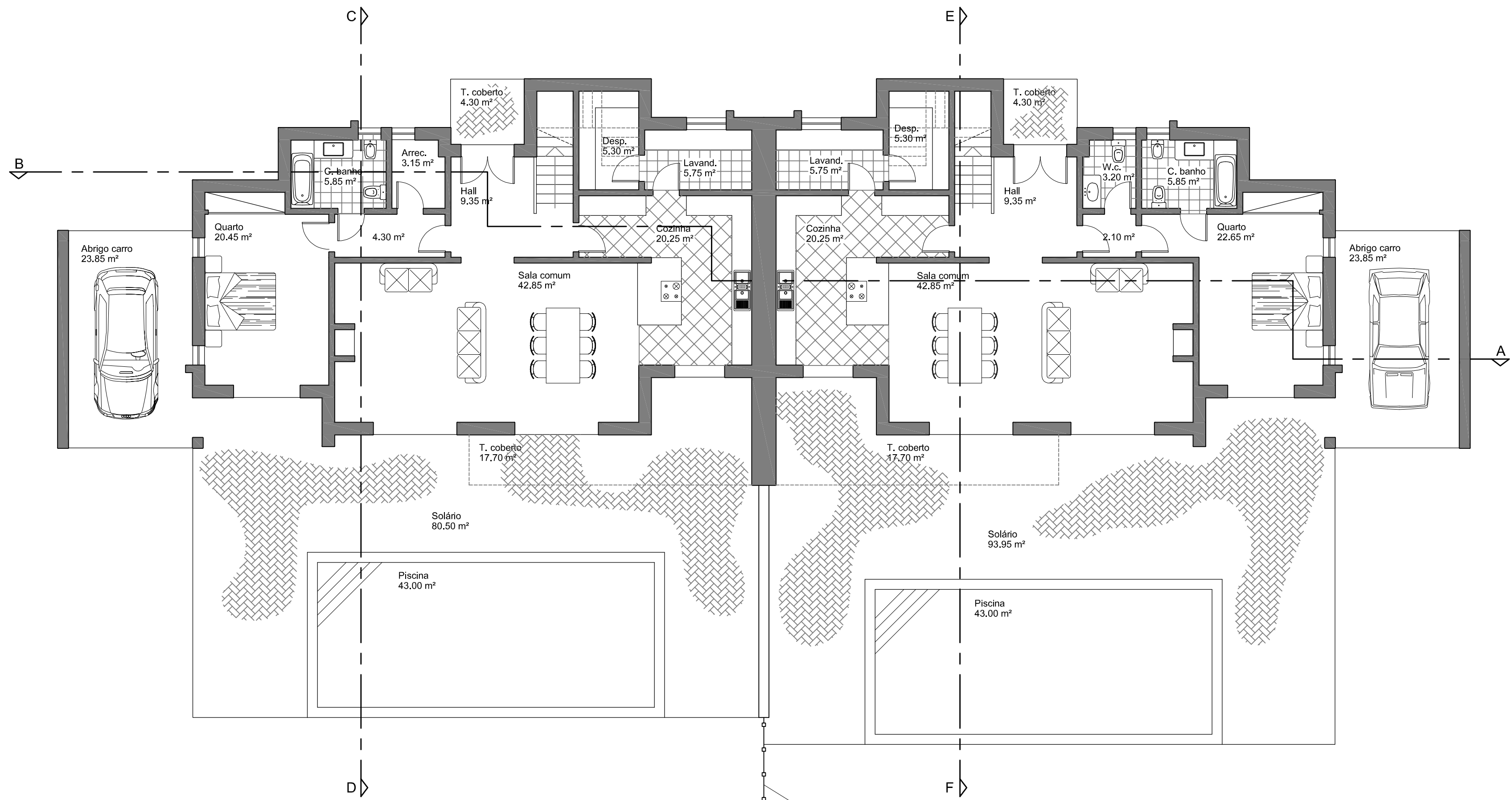
PLANTA DO R/CHÃO
